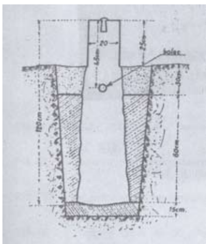
Kamień niwelacyjny
