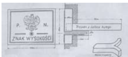
Reper tabliczkowy
