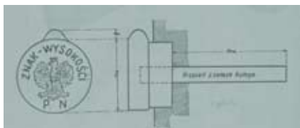
Bolec repera
